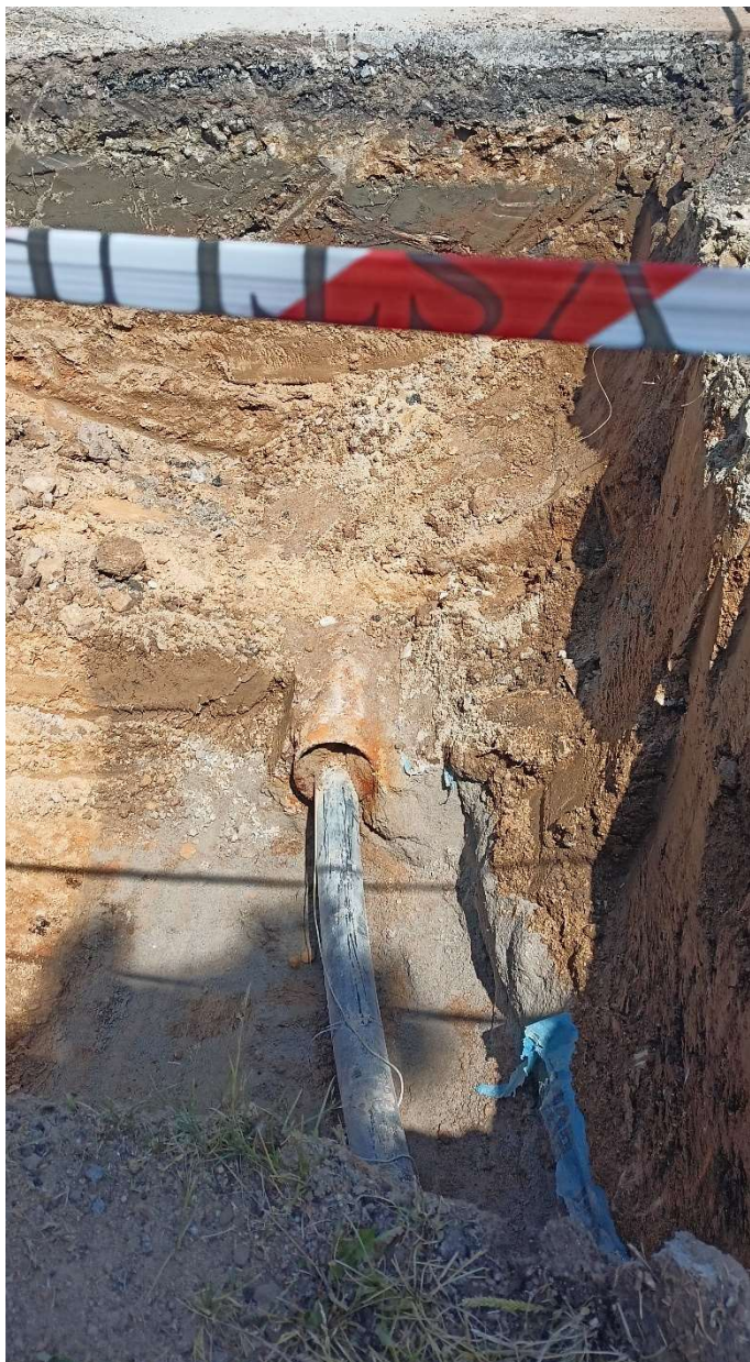
Stavba vodovodu ve Svatojánské ulici.
