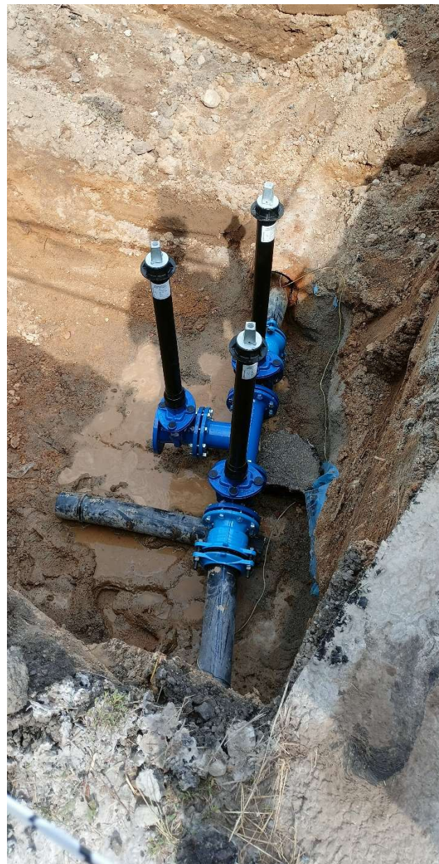
Stavba vodovodu ve Svatojánské ulici.
